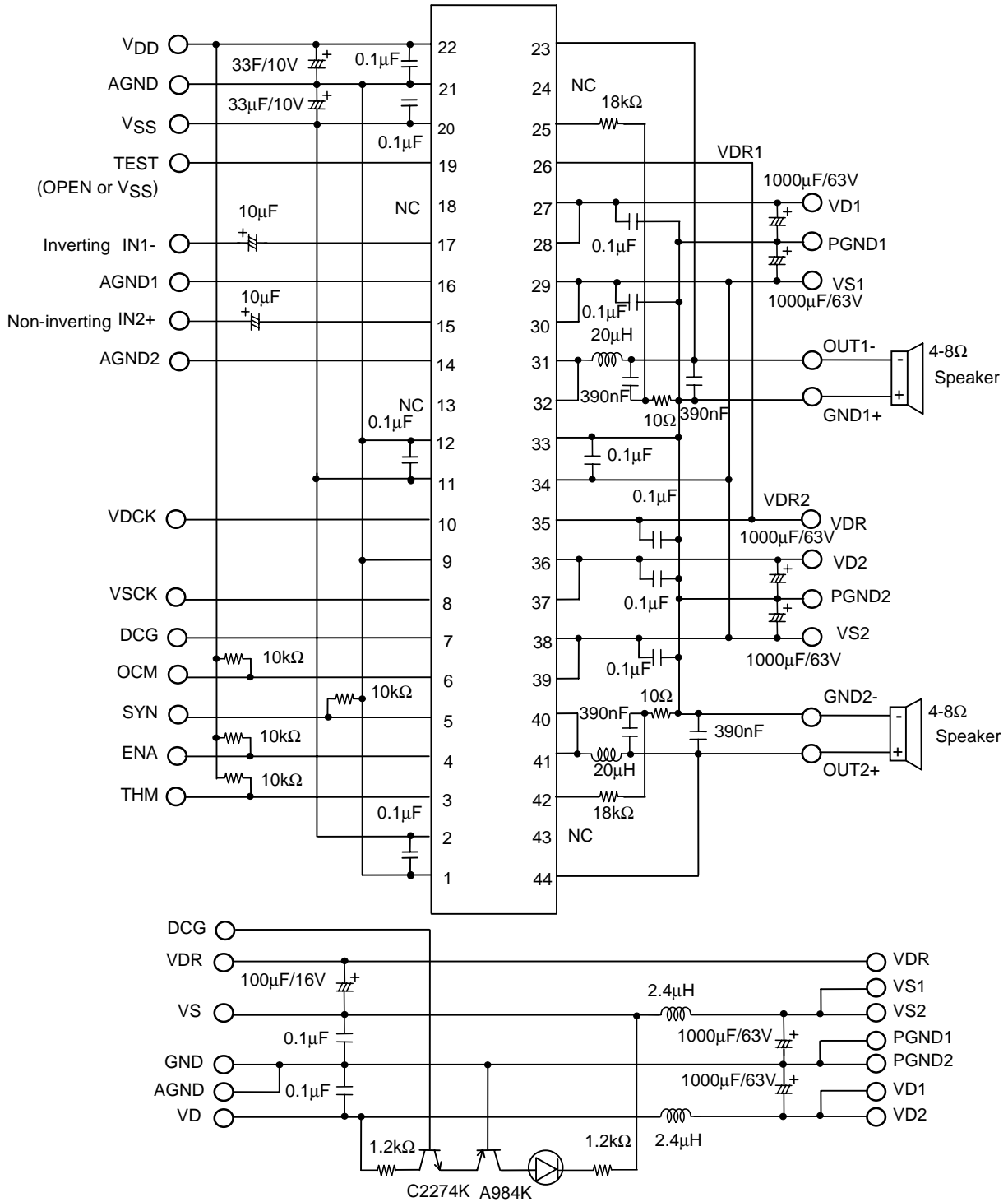
測定回路図
